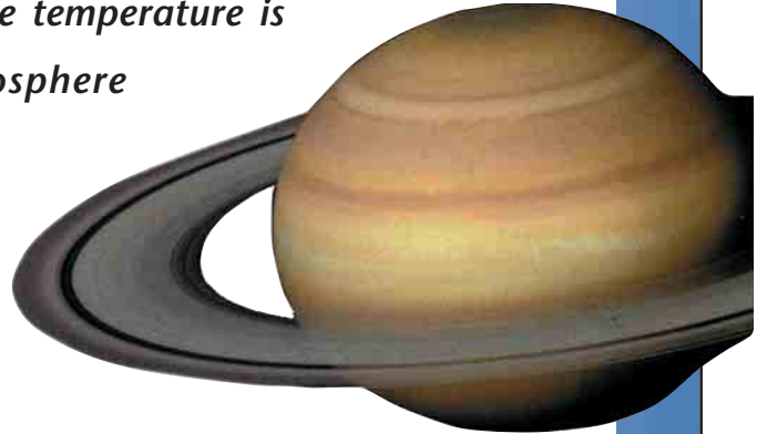
S aturn
